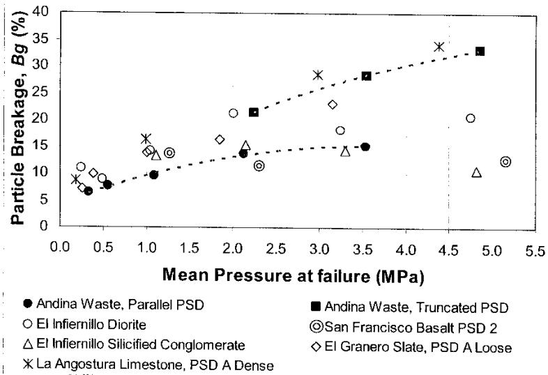
Figure 17 B_g Parameter variation
